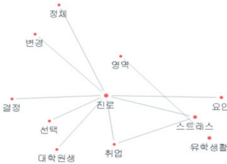
그림 13. Community 2
