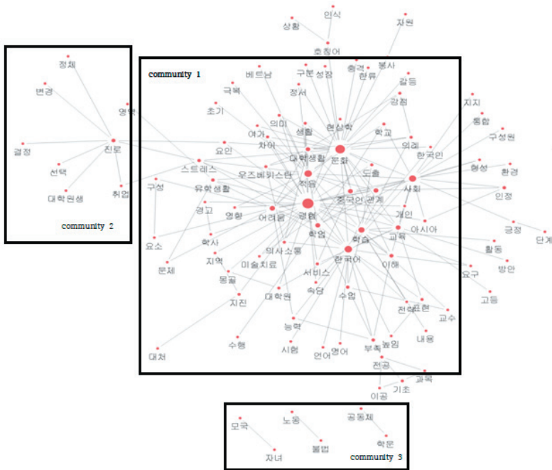
그림 11. 전체 시각화
